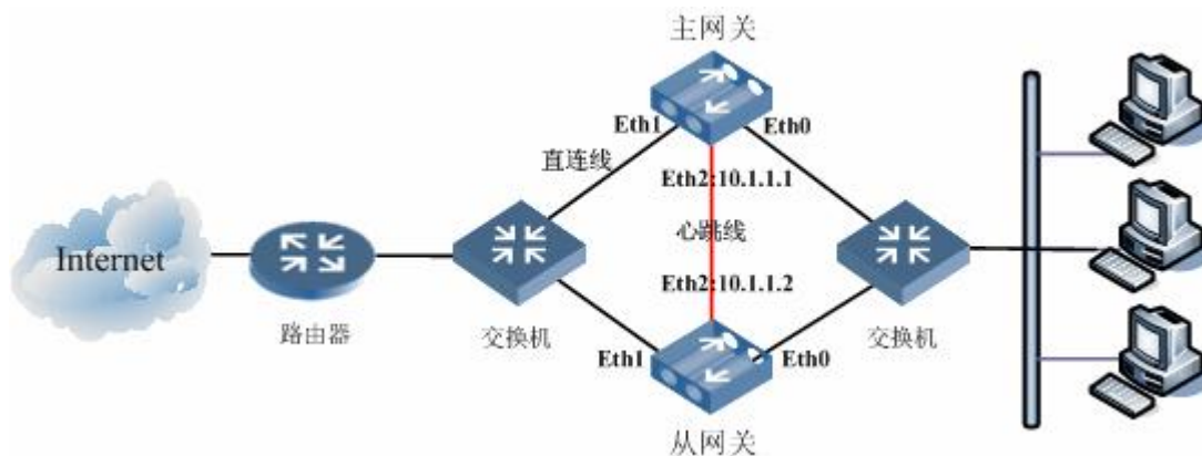
图 6-3 双机热备模式下的 VPN 应用
