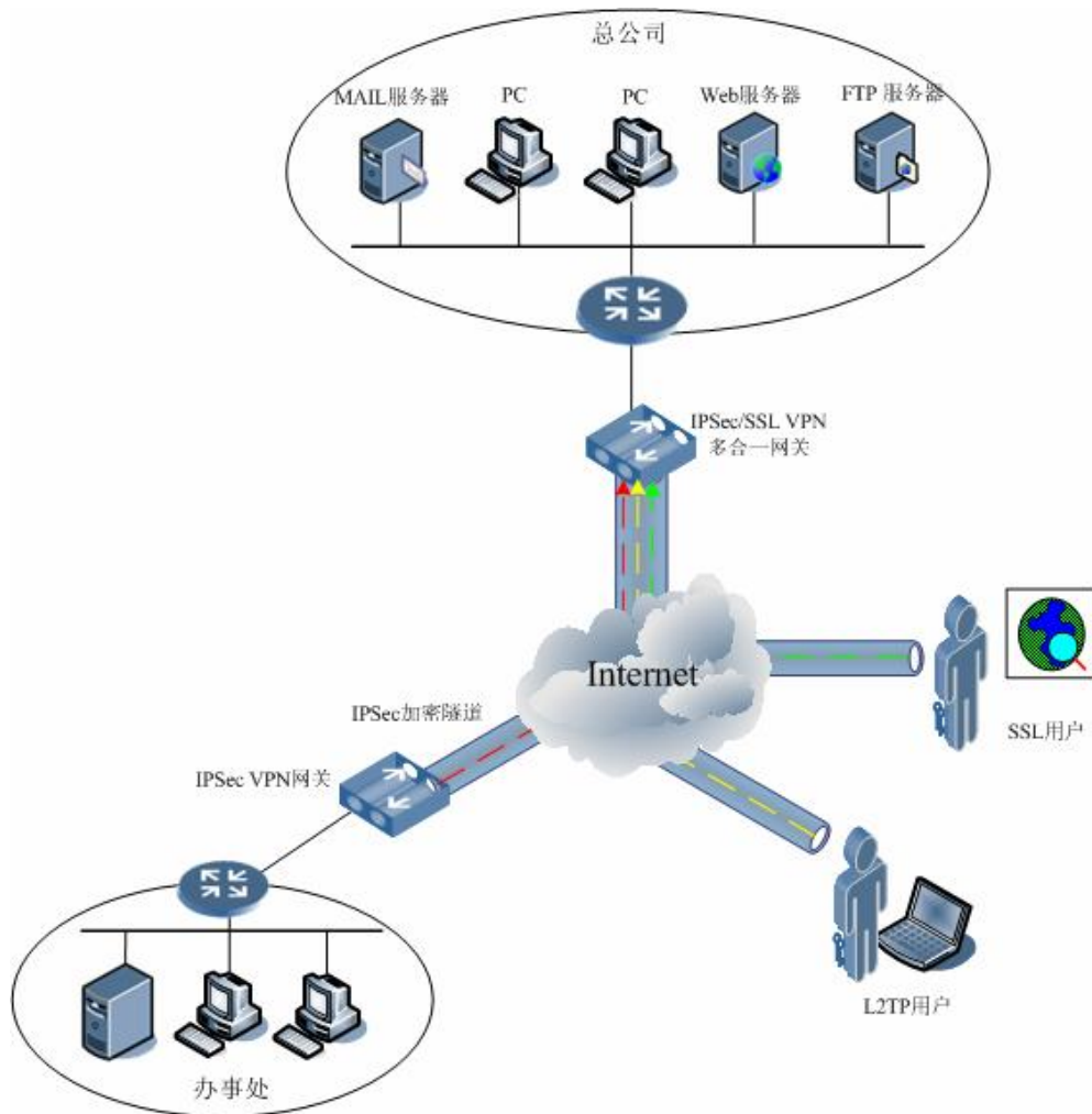
图 6-1 多种 VPN 综合应用示意图
