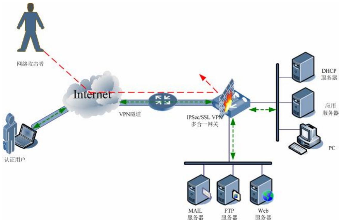
图 6-2 防火墙与 VPN 的综合应用
